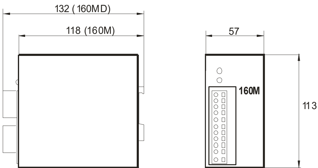
Rys. 2 Wymiary gabarytowe zasilaczy serii 160M/MD
