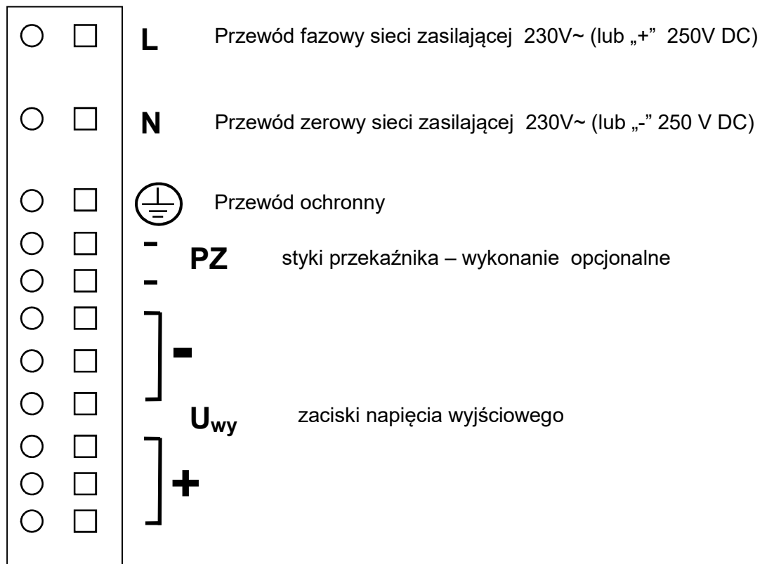
Złącze zaciskowe w zasilaczach serii 280SD
