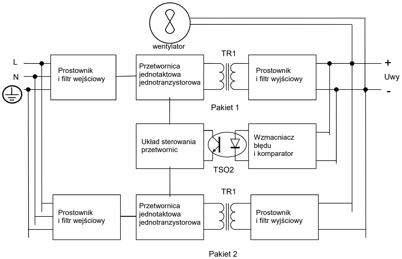
Rys. 2 Schemat blokowy zasilacza SPS-280SD
